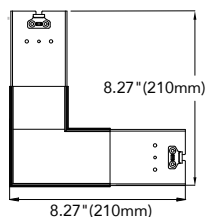
LLS(L-Shape)
